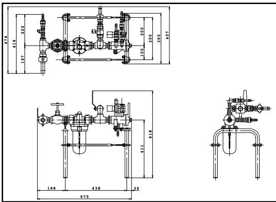
バルブスタンド概略寸法図
