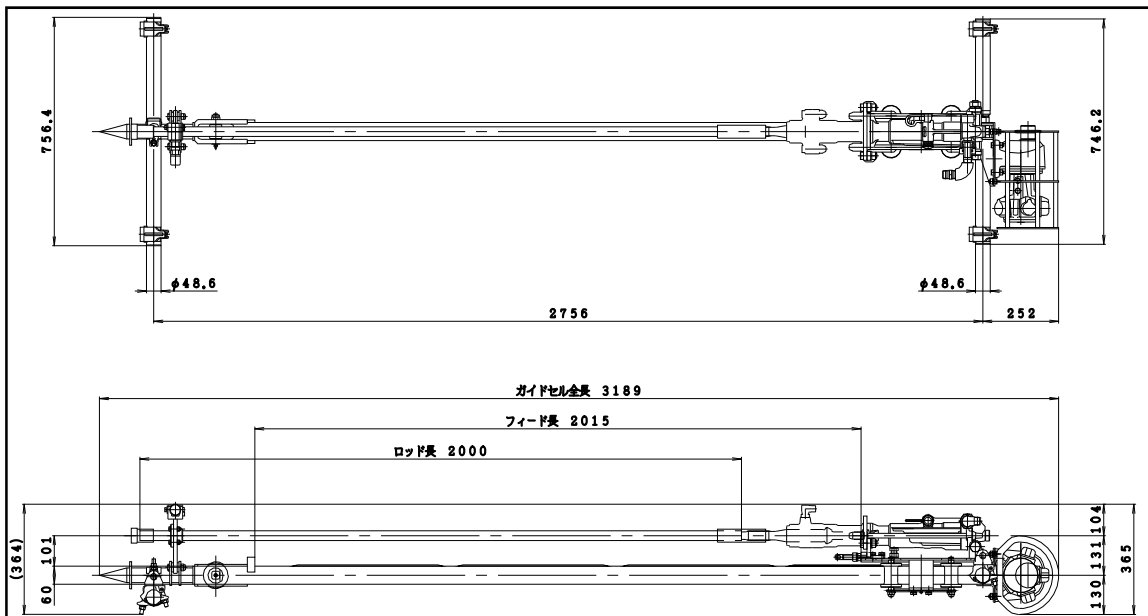
ガイドセル概略寸法図
